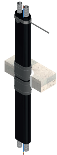
Solarleitung auch mit Elektrobegleitkabel
